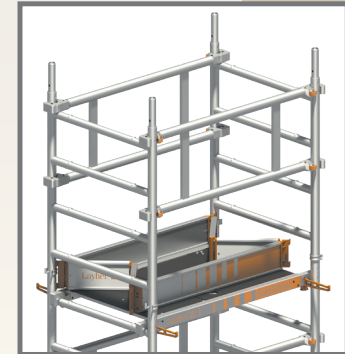
Detail Durchstiegsbrücke
